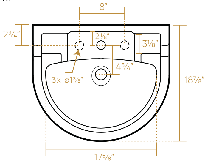
TOP
